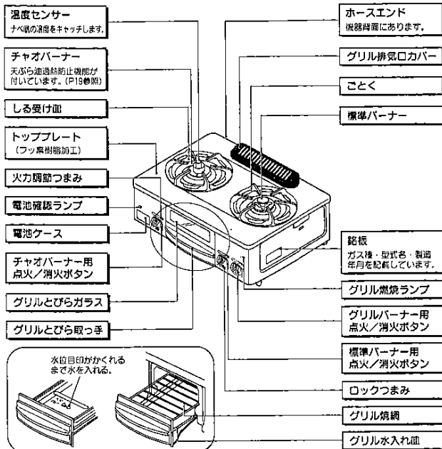
[グリルとびら部拡大図]
