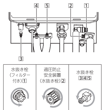
水抜き栓の位置 (各水抜き栓は、保温材などで見えにくいことがあります)
