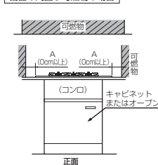
機器の周囲が可燃物の場合
