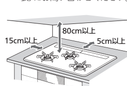
<可燃性の壁の場合>
