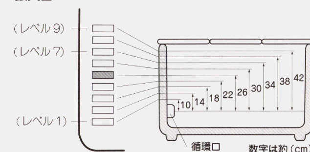
ふろ水位表示部 拡大図
