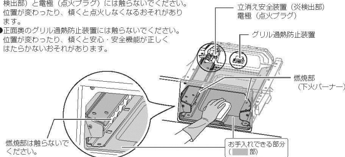
下火バーナー部拡大図
