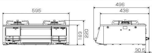
外形寸法図 (単位: mm)
