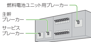
家庭用燃料電池対応分電盤
