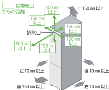
貯湯ユニット
