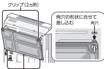
エアフィルターを3カ所の受け部にのせる
