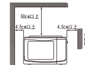
正面図
