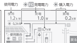
太陽光発電電力と発電電力と買電電力の使用割合
