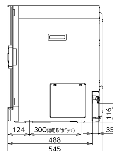
側面図
