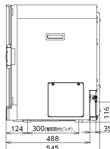
側面図
