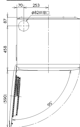
上面図
