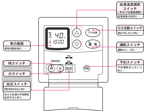
台所リモコン(036-0650型)[別売部品]
