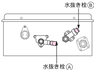
（ 機 器 底 面 ）
