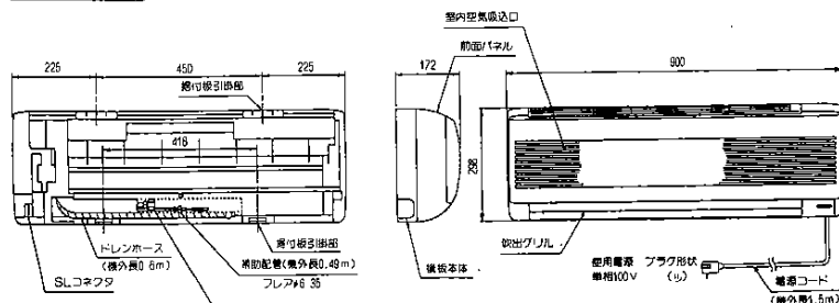
室内ユニット (48-506, 48-507)
