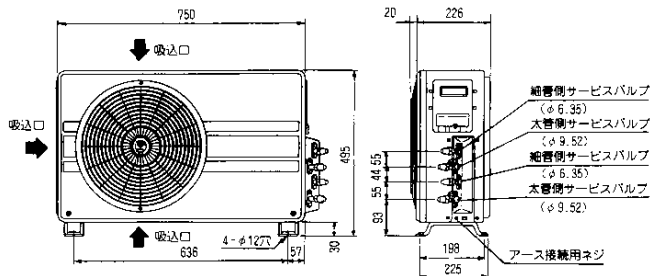
寸法図
