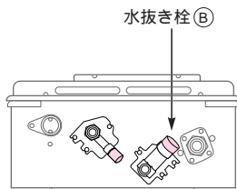
（機器底面）
