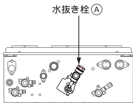
（機器底面）
