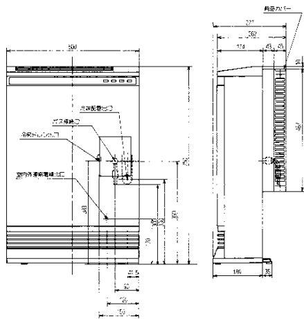
44-350型 ガスファンヒーターエアコン
