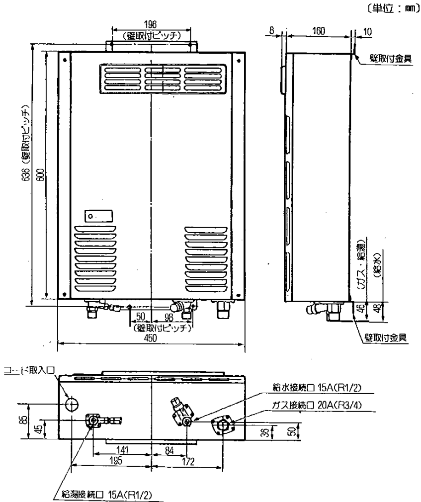
33-960型(壁掛設置タイプ)
