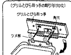
(グリルとびら取っ手の取り付けかた)
