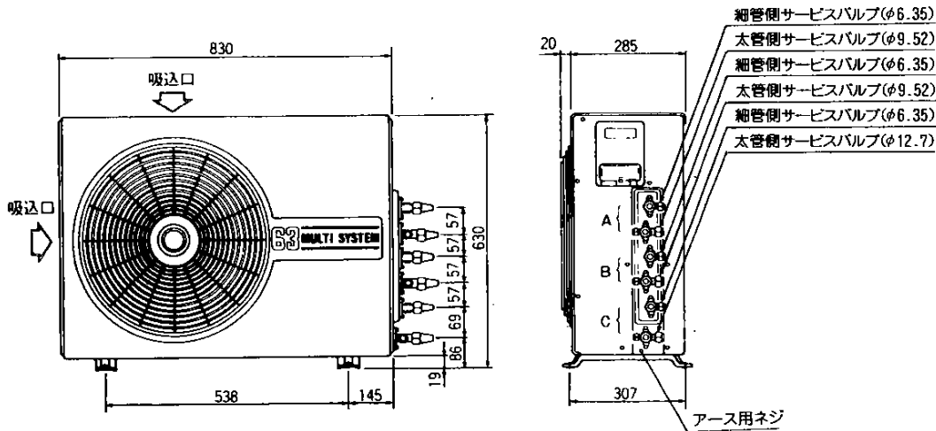
■冷房用室外機（3室マルチ型）04-278A型
