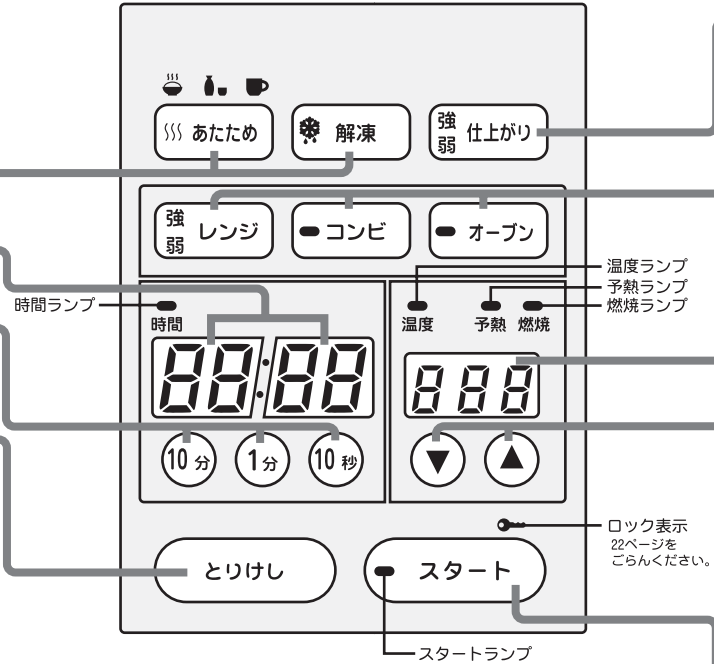
ガス高速オープンタイプ (114-H513型)
