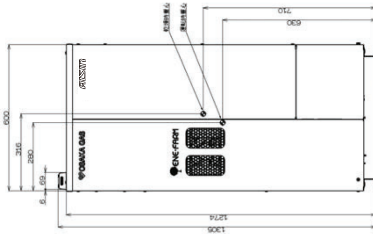
正面図
