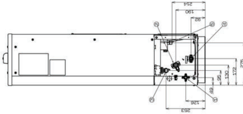
後面図
