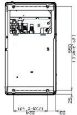
下面図
