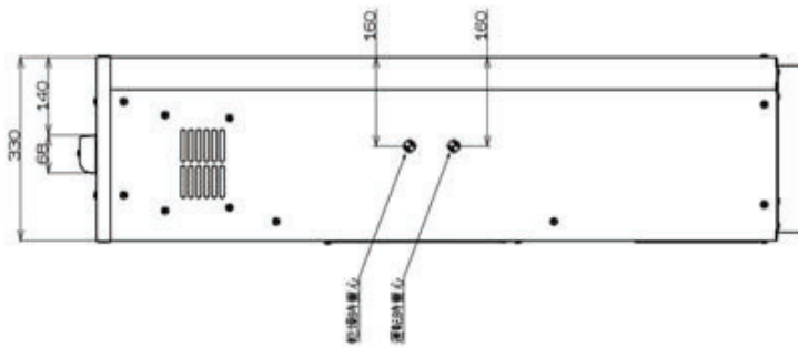
左側面図
