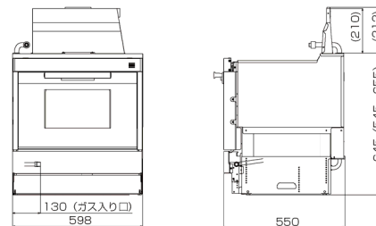
外形寸法図(単位: mm)
